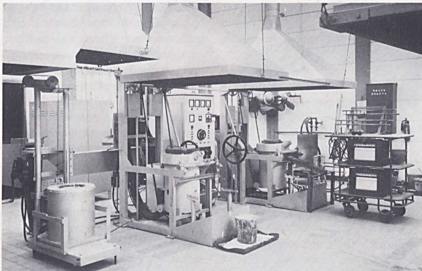
Batterij midden frequent-inductie ovens met regel- en meetapparatuur in de proefgieterij van het Gieterijcentrum.
