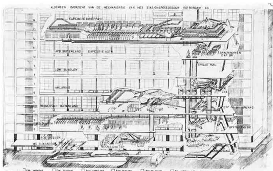
Overzichtstekening van het districtspostkantoor te Rotterdam
