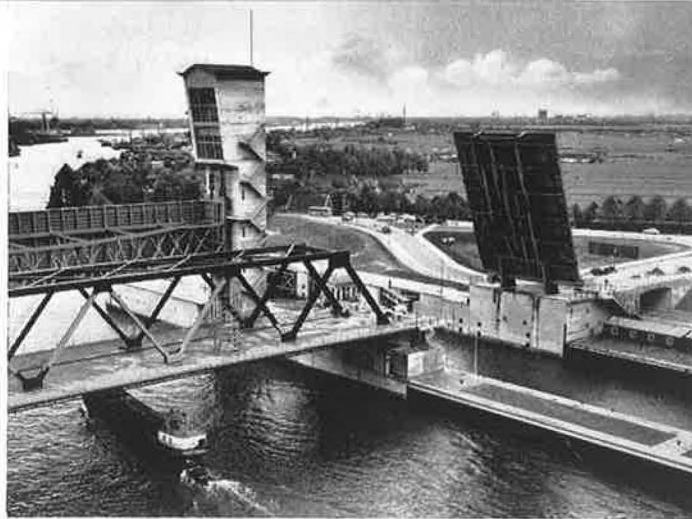
Rechts een schutsluis van 110 m kolklengete en daarnaast een afsluitbaar gedeelte van 80 m. De beweegbare brug en de vaste bruggen liggen 8½ m boven N.A.P. Links de vaste brug die door een 500 m lang viaduct met de Krimpenerwaard is verbonden. De schuiven die bij stormvloed naar beneden worden gelaten, wegen elk ca. 600.000 kg en zijn opgehangen in 45 m hoge torens.
